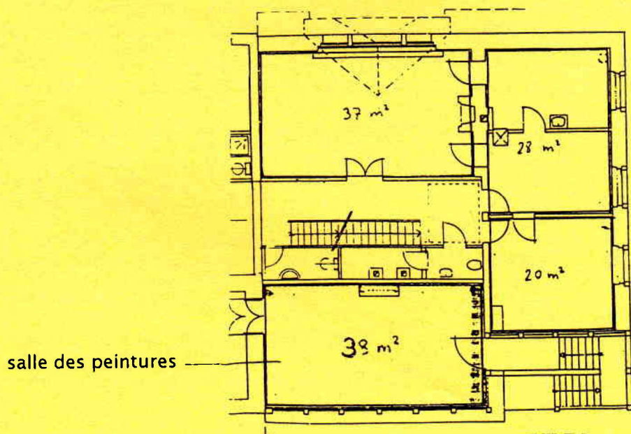
PLANS DU REZ et du 1er ETAGE
